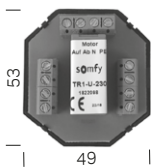
1-fach Trennrelais TR1 Art. Nr. TR1
